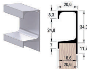
103419-PERFIL ALUM PUX 5047 18MM ANOD
