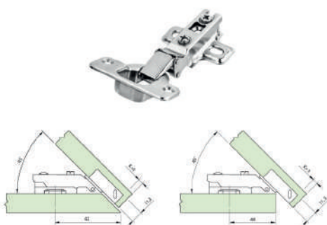
Dobradiça Ângulo -45°
