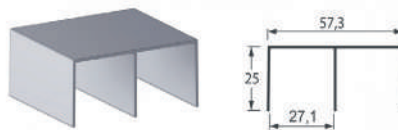
102026-PERFIL TRILHO SUP 2055 15MM ANOD 102032-PERFIL TRILHO SUP 2055 15MM INOX
