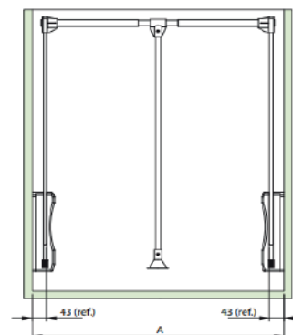
101852 - CABIDEIRO BASC 660-890 PRETO/CROMADO 101853 - CABIDEIRO BASC 890-1210 PRETO/CROMADO
