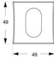
102254-FECHADURA P/PORTA PIVOTANTE STAM
