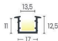
101984 - PERFIL ALUM LED 02 ANOD 6MT - ALTERNATIVA
