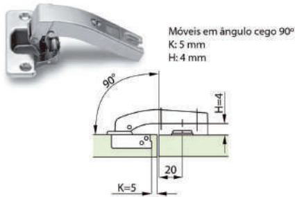
Dobradiça 90 ° ângulo cego
