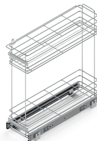
101800 - PORTA LATA CROMADO DUPLO CORREDICA TElesc INFERIOR A 490 X L160 X P 460
