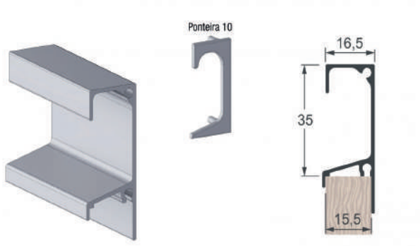
101979-PERFIL ALUM PUX 5046T 15MM ANOD 101980-PERFIL ALUM PUX 5046T 15MM INOX
