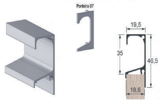
101982-PERFIL ALUM PUX 5047T 18MM ANOD 101983-PERFIL ALUM PUX 5047T 18MM INOX
