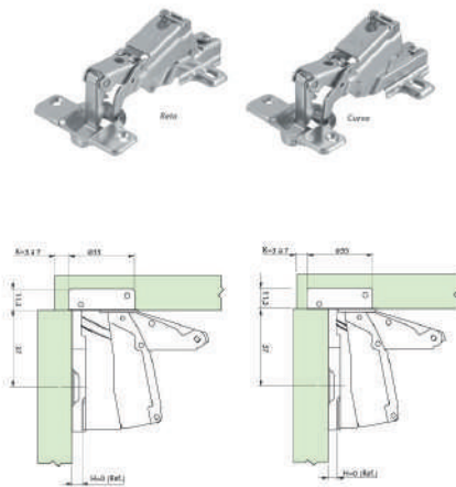
Dobradiça 165°
