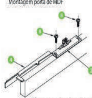
Montagem do acionador utilizando o gabarito de instalação
