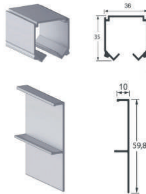
103749 - PERFIL ACABAMENTO 2092 ANOD
