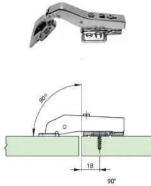
Dobradiça 90 °
