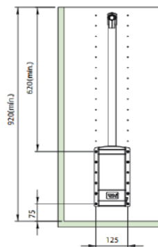
101852 - CABIDEIRO BASC 660-890 PRETO/CROMADO 101853 - CABIDEIRO BASC 890-1210 PRETO/CROMADO
