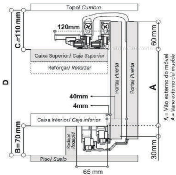
103846-TRILHO INFERIOR AL RM-264 DOMINUS ANOD 6MT ROMETAL
