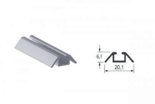
102033-PERFIL TRILHO INF 2051 ANOD 102034-PERFIL TRILHO INF 2051 INOX
