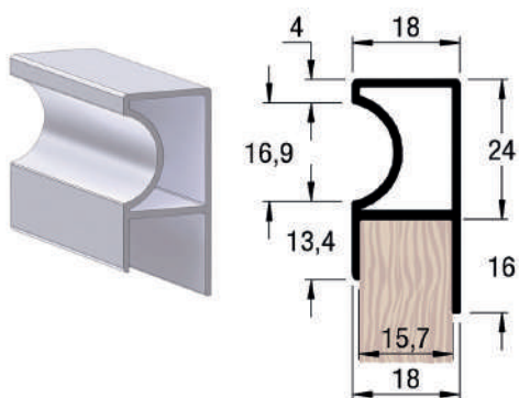
101991-PERFIL ALUM PUX 4003 15MM ANOD
