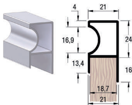
101992-PERFIL ALUM PUX 4004 18MM ANOD
